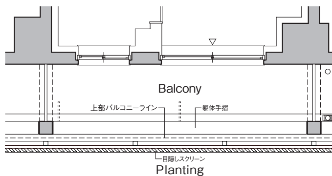
■ 119号室部分図
