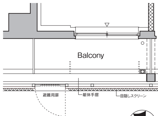
■ 113号室部分図
