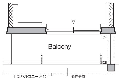
■ 104号室部分図
