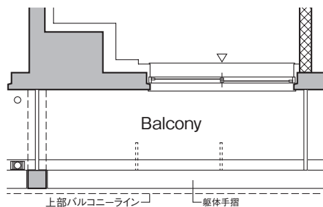
■ 105号室部分図
