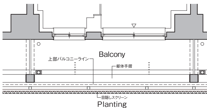
■ 118号室部分図
