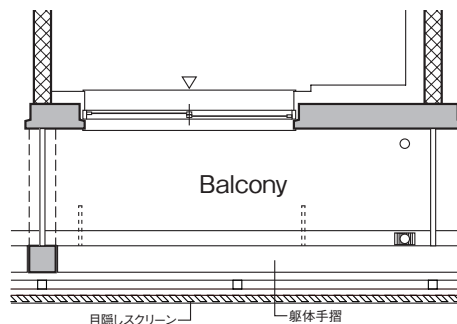
■ 115号室部分図
