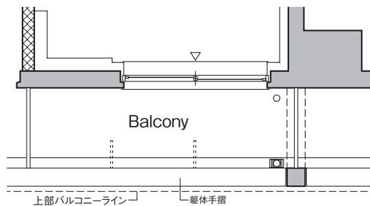
■ 106号室部分図
