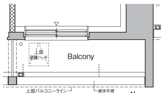
■ 122号室部分図
