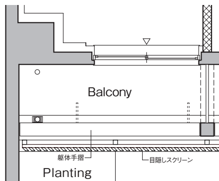
■ 116号室部分図
