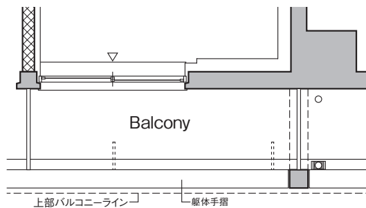
■ 110号室部分図
