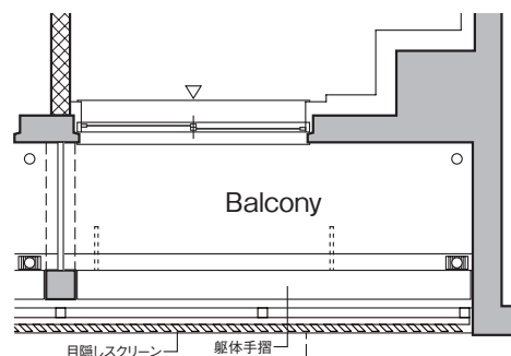
■ 112号室部分図
