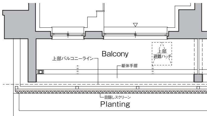
■ 120号室部分図
